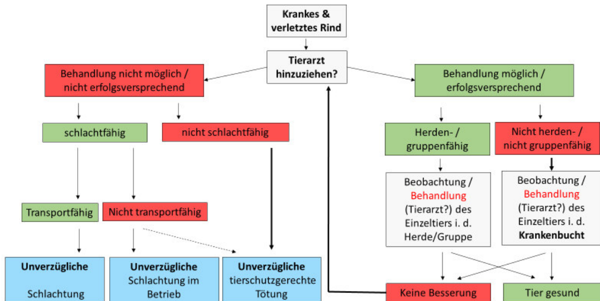
Abb.: 20 Entscheidungsbaum
